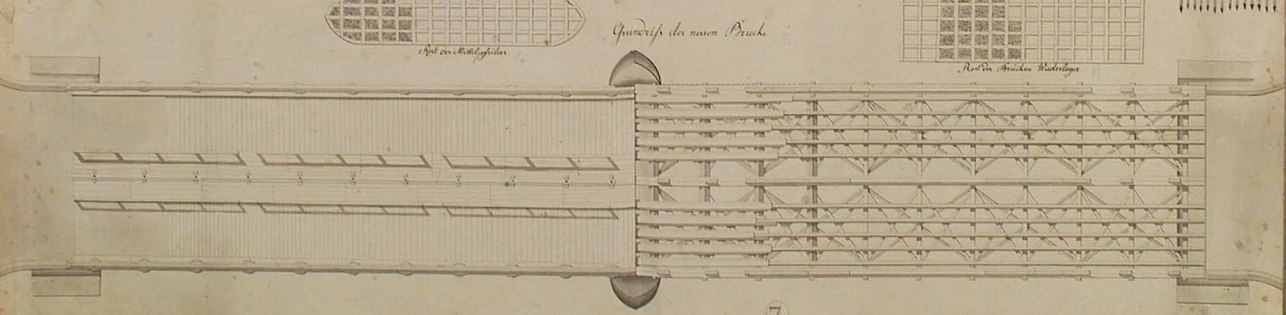
Ansicht für den Querschnitt und die Längs Profil des neuen Brücke
